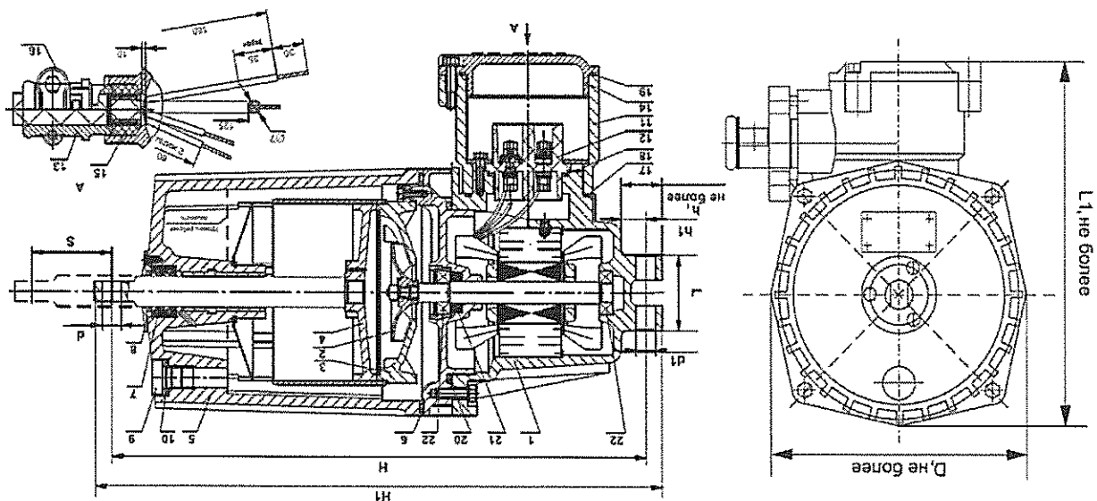
Рис. 1. Габаритные и присоединительные размеры ТЭ-150РВ
