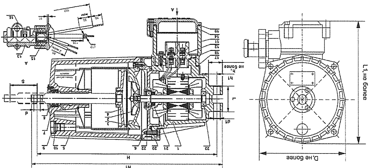
Рис.1. Габаритные и присоединительные размеры ТЭ-80МРВ
